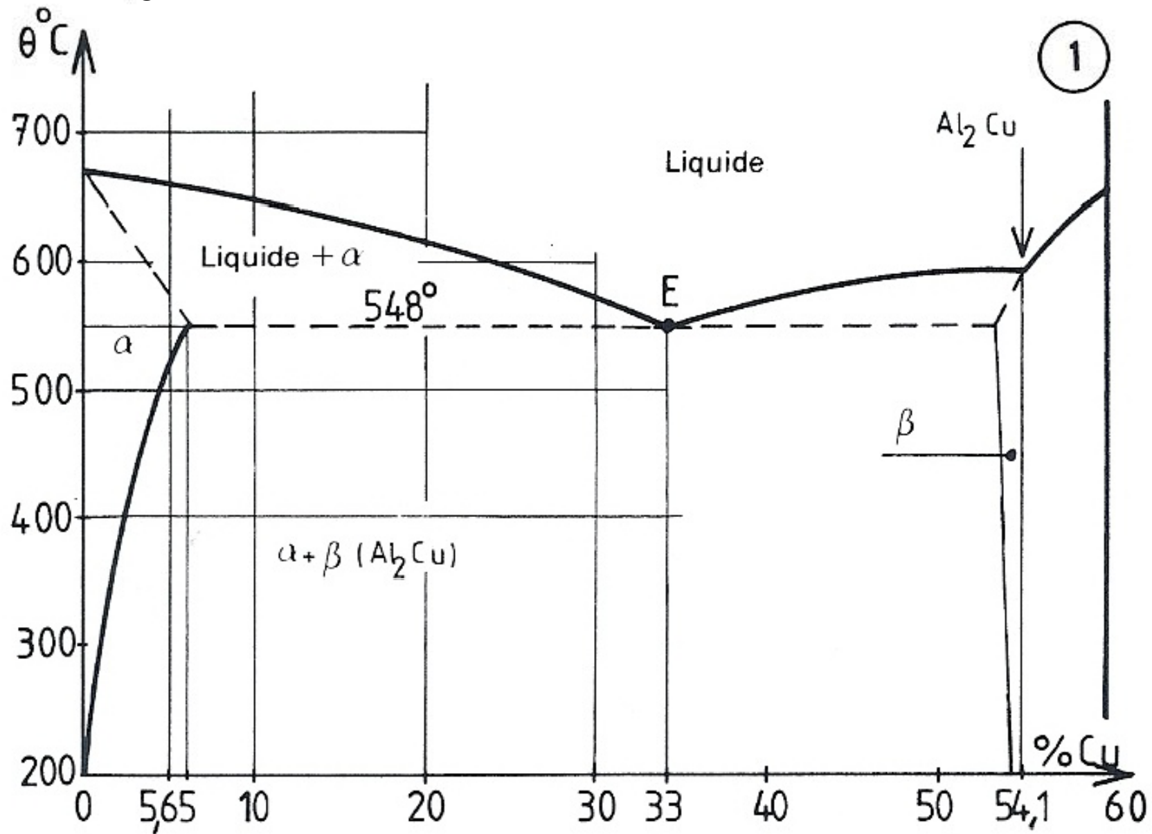
Diagramme d'équilibre Al. Cu.
