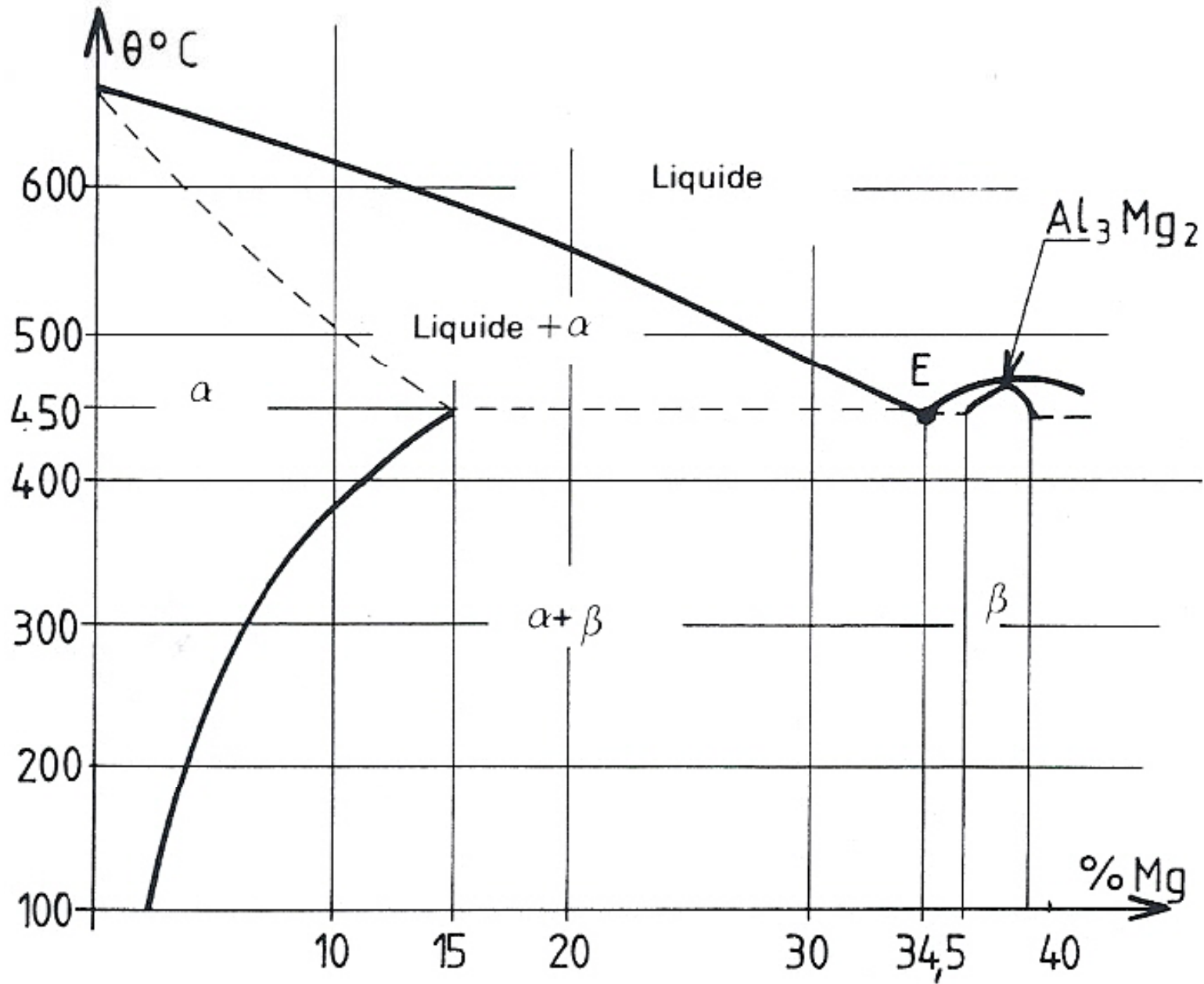
Diagramme d'équilibre Aluminium Magnésium
