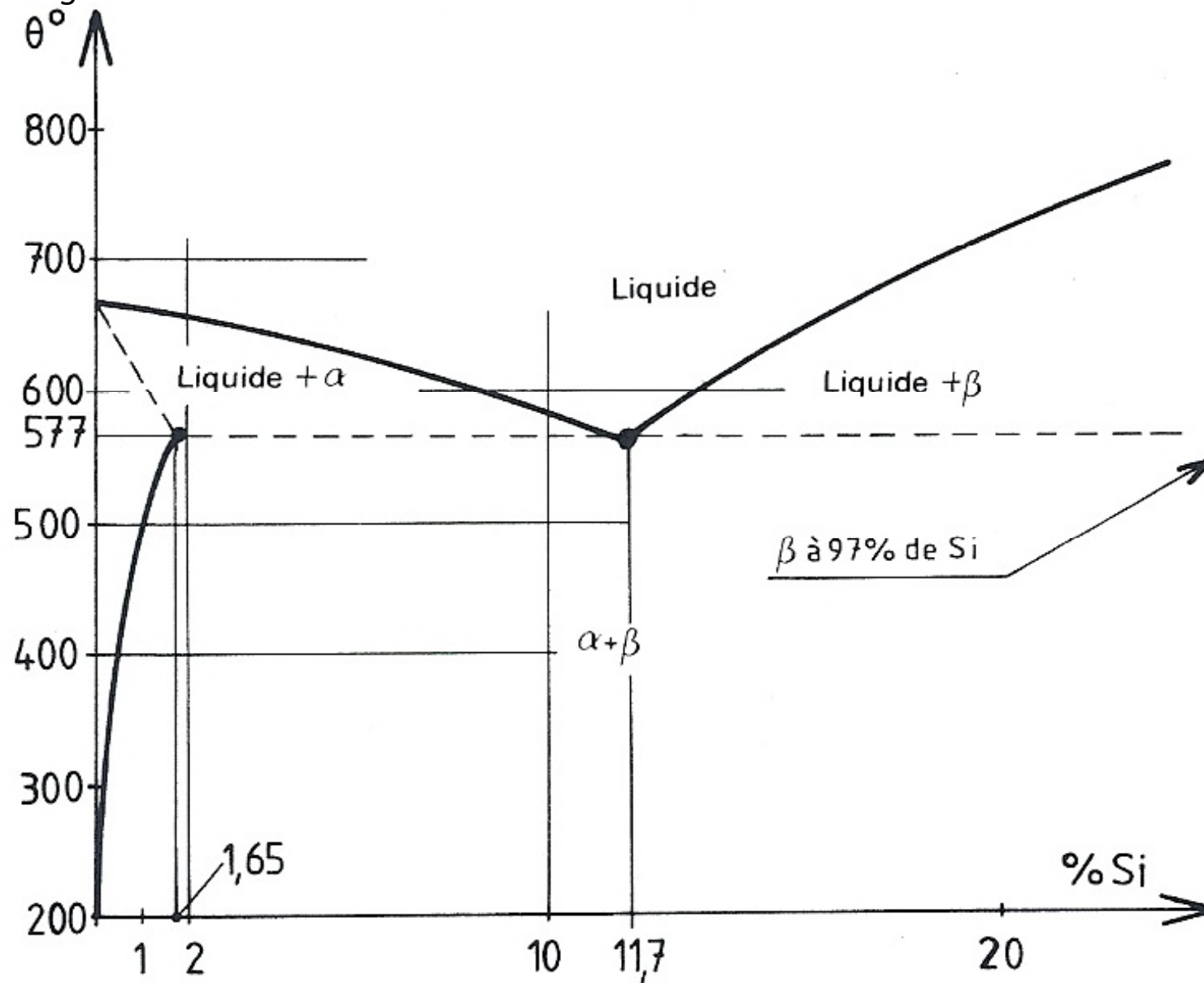
Diagramme d'équilibre Al. Si.
